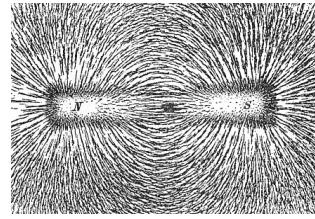
aimant permanent (photographie d'arrangement de la limaille de fer autour de l'aimant) Les lds vont du nord vers le sud
